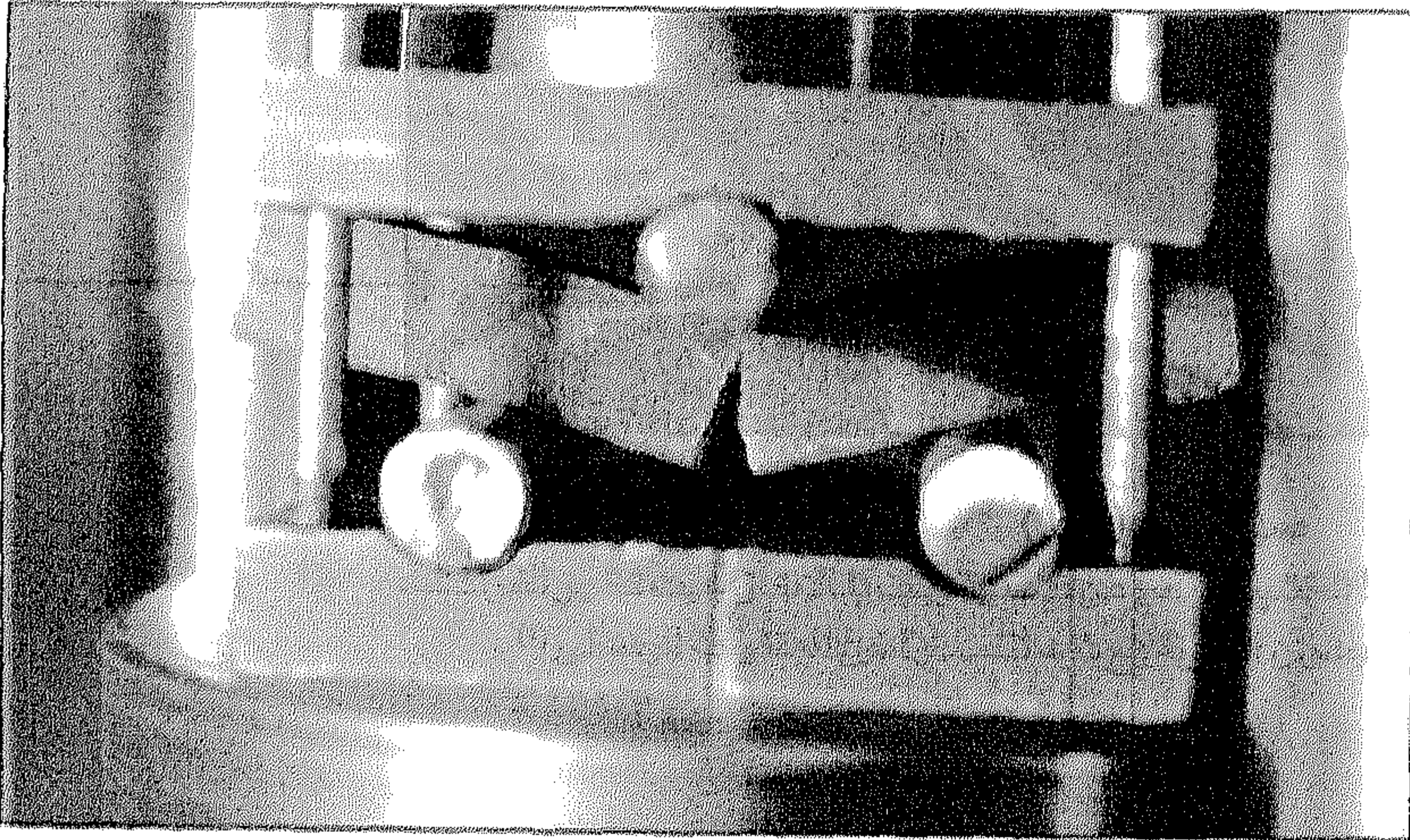
العينة (١٧) عند ضغط انحناء ١٥٥ كجم/سم ٢
